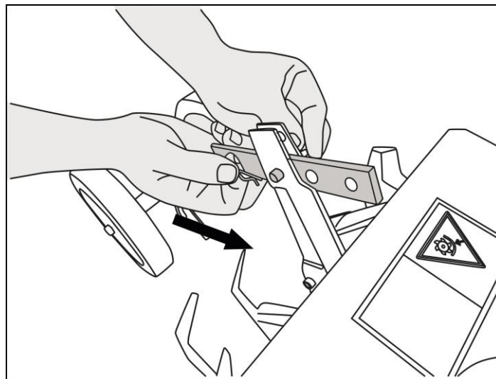
Рис. 6. Установка сошника
