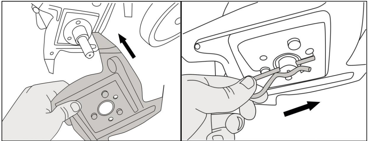
Рис. 5. Установка фрез
